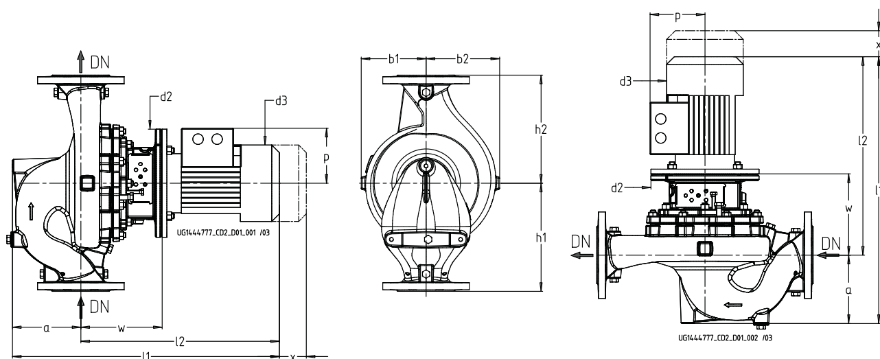
Габаритные размеры насоса
