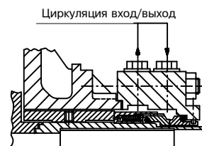
Торцовое уплотнение с воздушным охлаждением теплообменника
