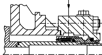
Торцовое уплотнение одинарного действия, без охлаждения
