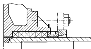
Набивка сальникового уплотнения неохлаждаемое уплотнение
