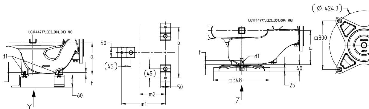
Габаритные размеры крепления к фундаменту
