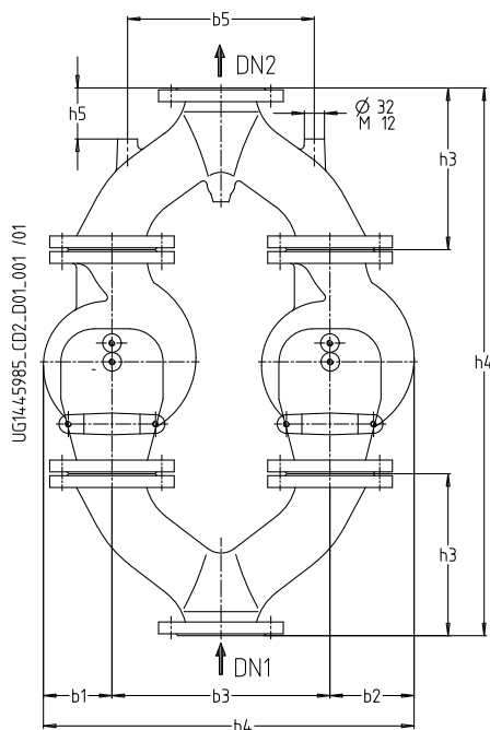
Габариты коллекторов
