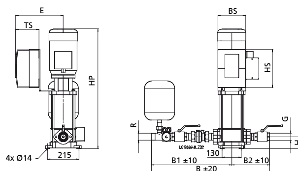
Няа-Solo DV с Movitec 6B и 10B
