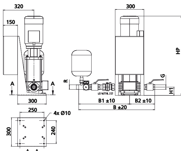
Няа-Solo D с Movitec 6B и 10B
